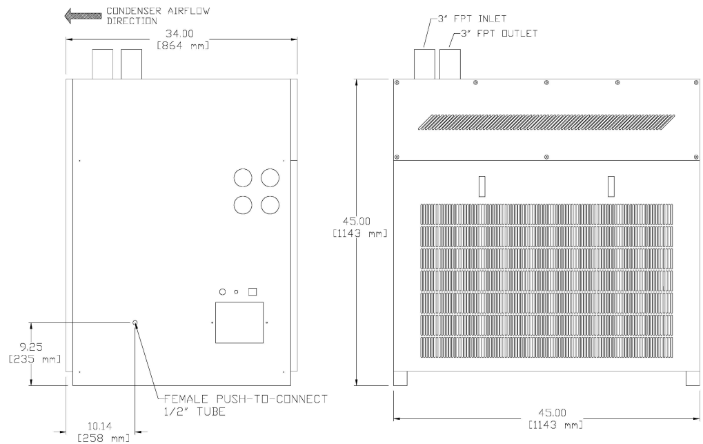
MODEL VF-600 DIMENSIONS
